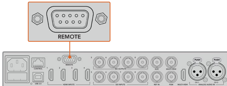
Uzaktan kumandalı bir kafayı, arka panelde 'remote' olarak etiketli RS-422 portu üzerinden ATEM switcher'inize bağlayın.
