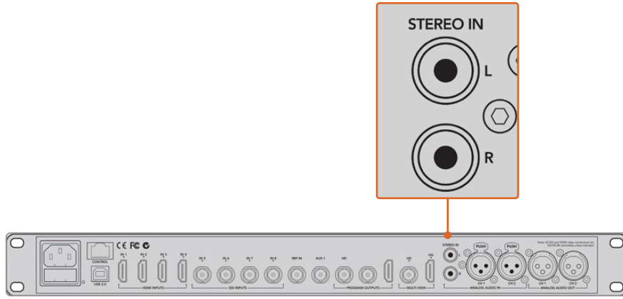
Harici HiFi sesini, RCA girişleri üzerinden switcher'inize bağlayın.
