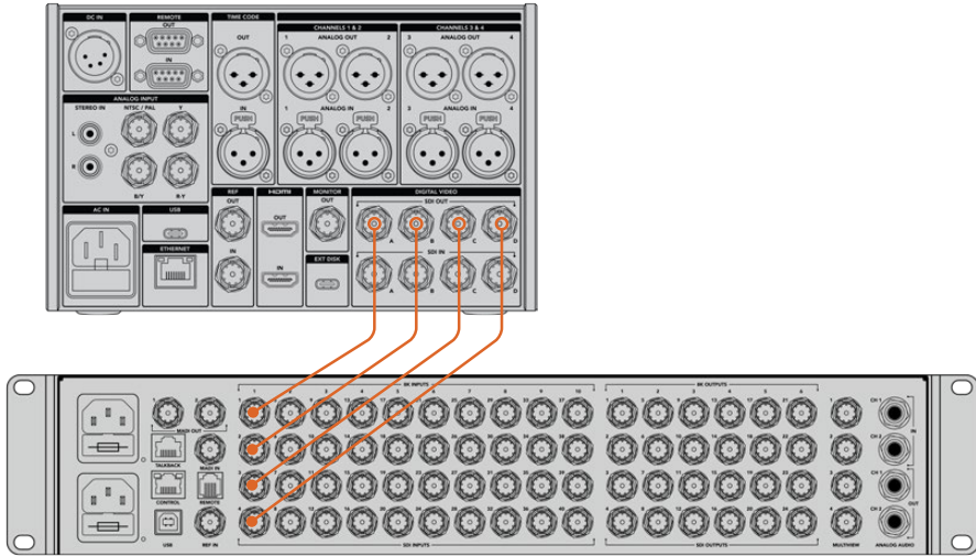
Bir HyperDeck Extreme 8K HDR'nin, 8K quad link SDI çıkışının, bir ATEM Constellation 8K'nın SDI girişine bağlanması.
