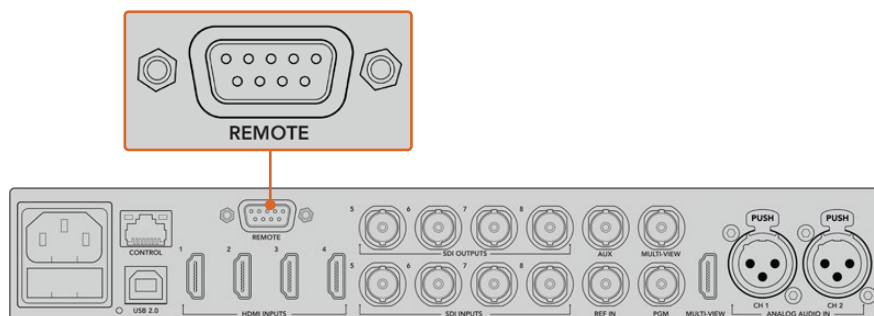
Connetti una testa remota allo switcher tramite la porta RS-422
