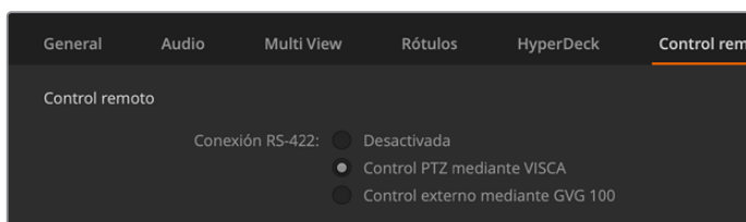
Opciones del puerto RS-422
