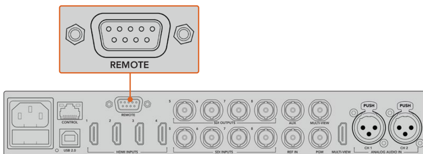
Для подключения панорамной головки используют порт RS-422 с маркировкой Remote на задней панели ATEM
