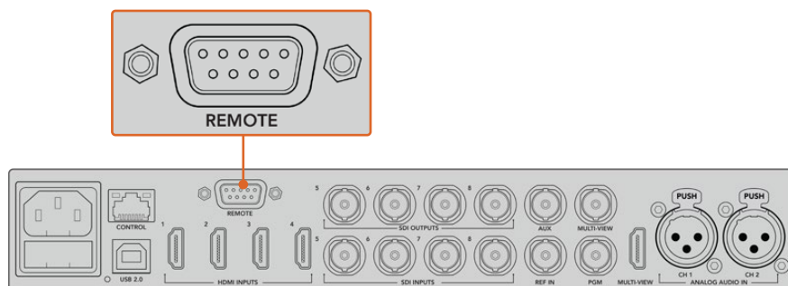
Conecte a cabeça remota ao seu switcher ATEM através da porta RS-422 rotulada “Remote” no painel traseiro.
