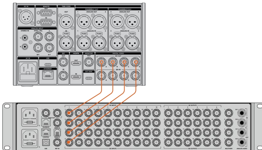
将HyperDeck Extreme 8K HDR的8K四链路SDI输出连接到ATEM Constellation 8K的SDI输入上。
