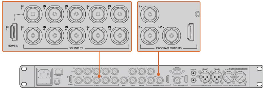
Blackmagic Studio Camera를 ATEM 스위처의 SDI 입력에 연결합니다.
