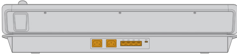
ATEM 2 M/E Advanced Panel arka bağlantıları
