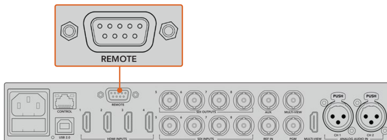
Schließen Sie einen Remotehead an den mit REMOTE gekennzeichneten RS-422-Port hinten am Mischer an
