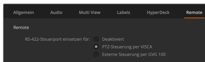
Steuern des RS-422-Remote-Ports über die Einstellungen „Deaktiviert“, „VISCA“ oder „GVG“
