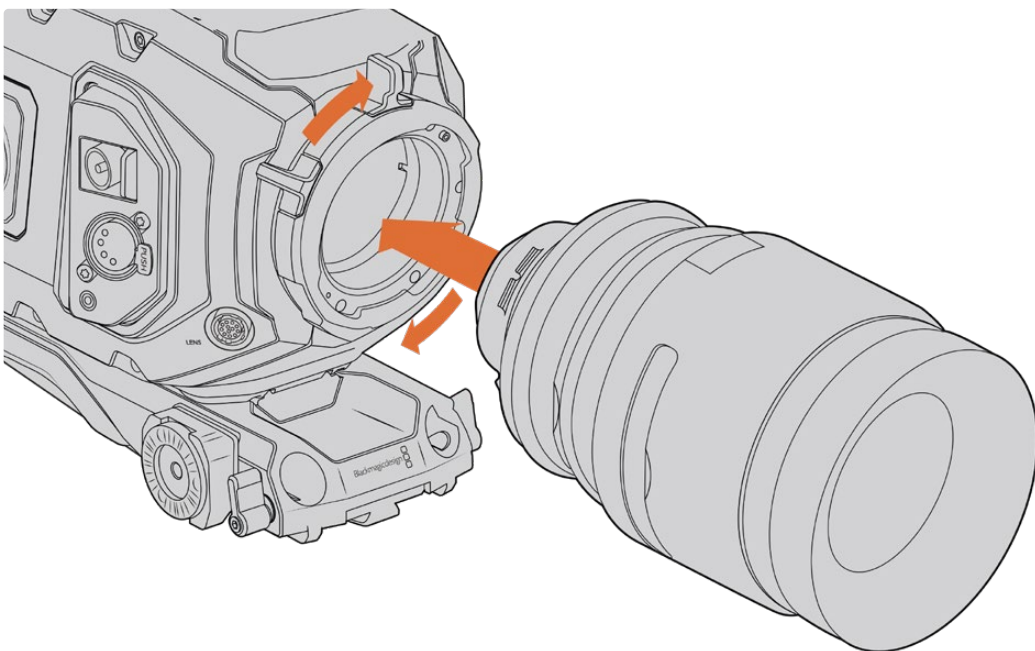
PLレンズをBlackmagic URSA Mini PLおよびURSA Mini Pro 12Kに装着/取り外し
