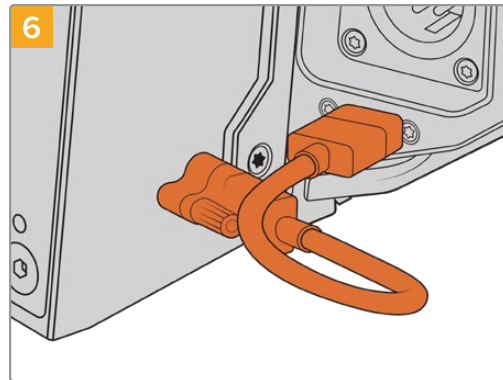
6 Mini Recorder의 USB-C 케이블을 URSA Mini Pro 12K 뒷면에 있는 USB-C 데이터 포트에 연결하세요. 손가락이나 2mm 육각 드라이버를 사용해 잠금 커넥터를 조이세요. URSA Mini Pro 4.6K G2를 사용할 경우, 길이가 긴 USB-C 케이블을 사용하여 CFast 슬롯 위에 있는 USB-C 포트에 연결하세요.
