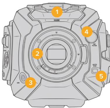
URSA Mini Pro 4.6K 모델
