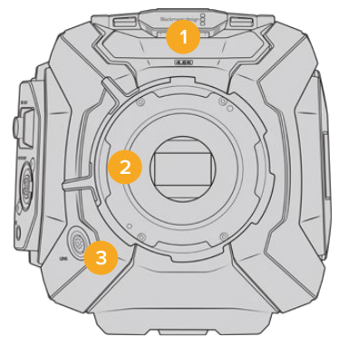
URSA Mini PL 모델
