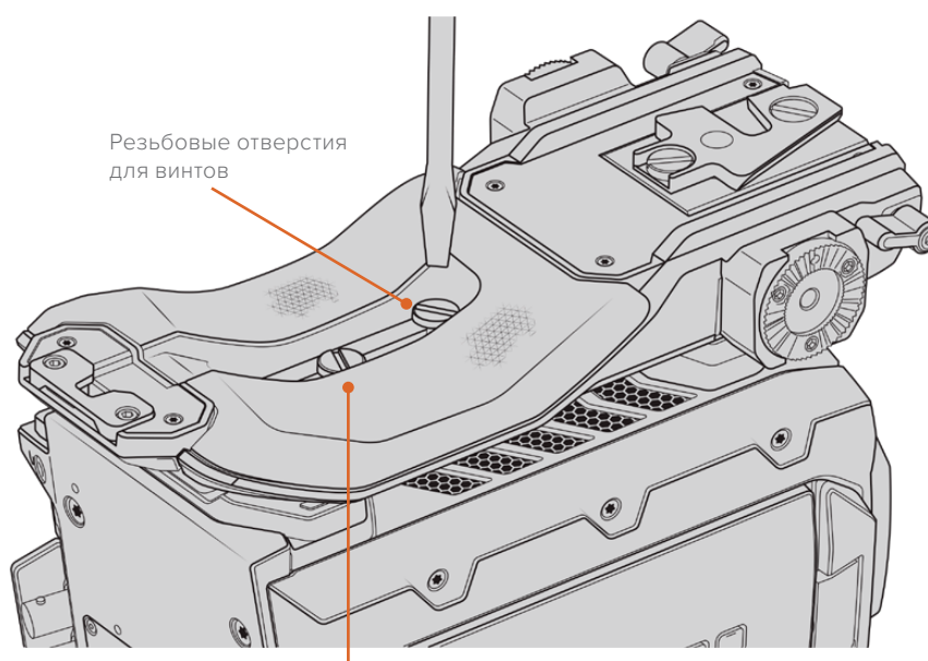
Два винта 1/4 дюйма для опорной пластины
