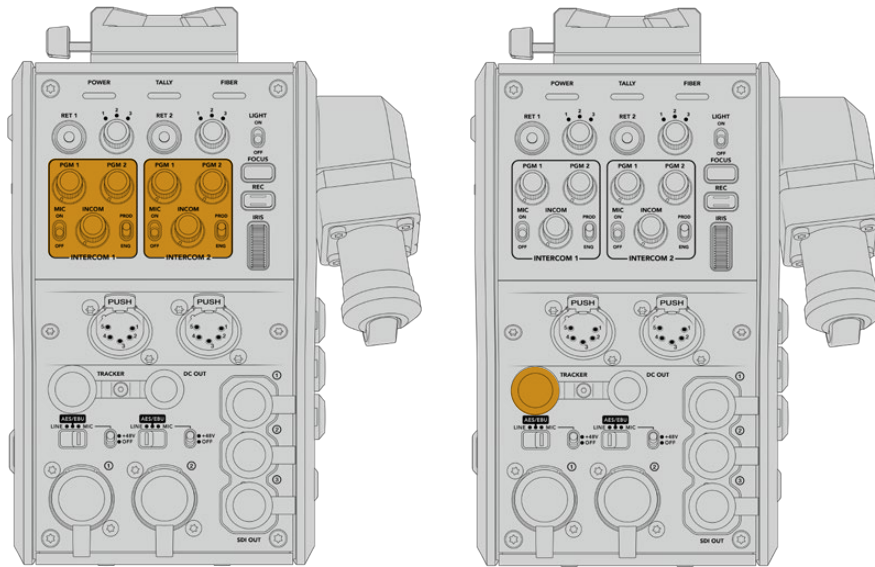
토크백 오디오 레벨 믹싱용 인터페이스 커넥터
