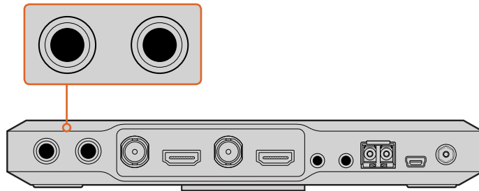
外部オーディオ機器をTRSコネクタで接続。
