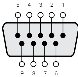
RS-422 원격 핀 연결
