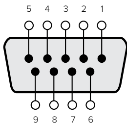
RS-422-Stiftverbinder zur Fernsteuerung
